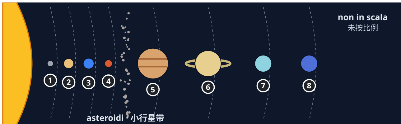
Gli otto pianeti in ordine di distanza dal Sole (dimensioni e distanze non in scala). 按与太阳距离排列的八大行星（大小和距离都未按比例）。
